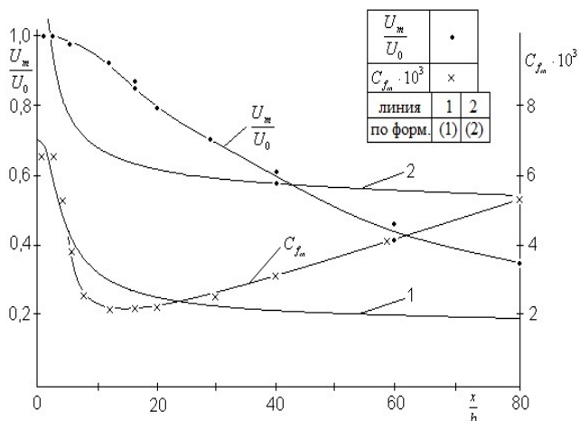
Рисунок 4 – Изменение коэффициента сопротивления трения на торцевой стенке при \lambda = 4, U_0 = 30 \text{ м/с}
